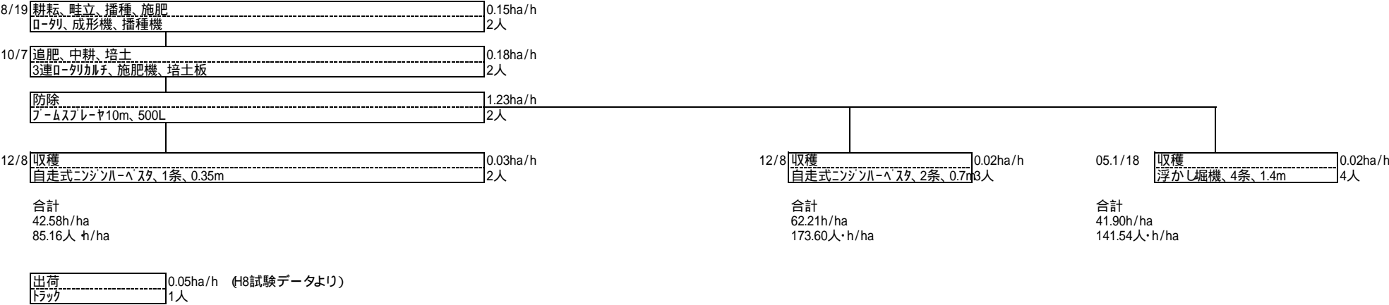
諫早湾干拓地におけるニンシン機械化体系
